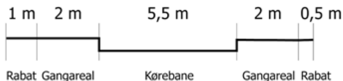
Vejprofil Kalvøvej
